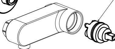
Ecrou de fixation 08HJA01
